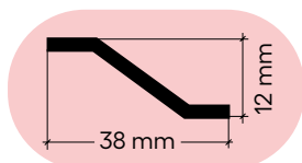
Perfil / Section
