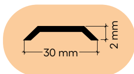
Perfil / Section
