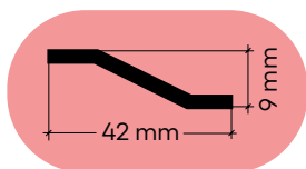
Perfil / Section
