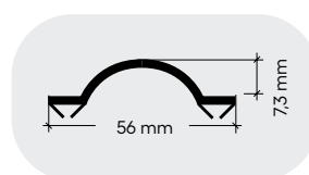
Perfil / Section
