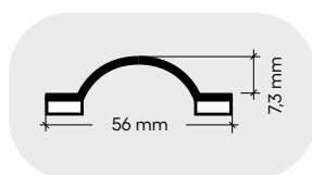
Perfil / Section
