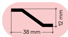
Perfil / Section
