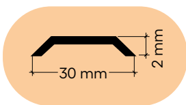
Perfil / Section
