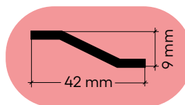
Perfil / Section
